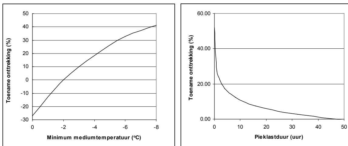
Figuur 4: Toename van het mogelijk te onttrekken vermogen (watt/meter) in relatie tot de gekozen toegelaten minimum temperatuur (links) en pieklastduur (rechts). Uitgangspunt is het temperatuurcriterium van -2\text{ }^{\circ}\text{C} (d.w.z.: linker grafiek bij 0\text{ }^{\circ}\text{C} 25% minder watt/meter ten
